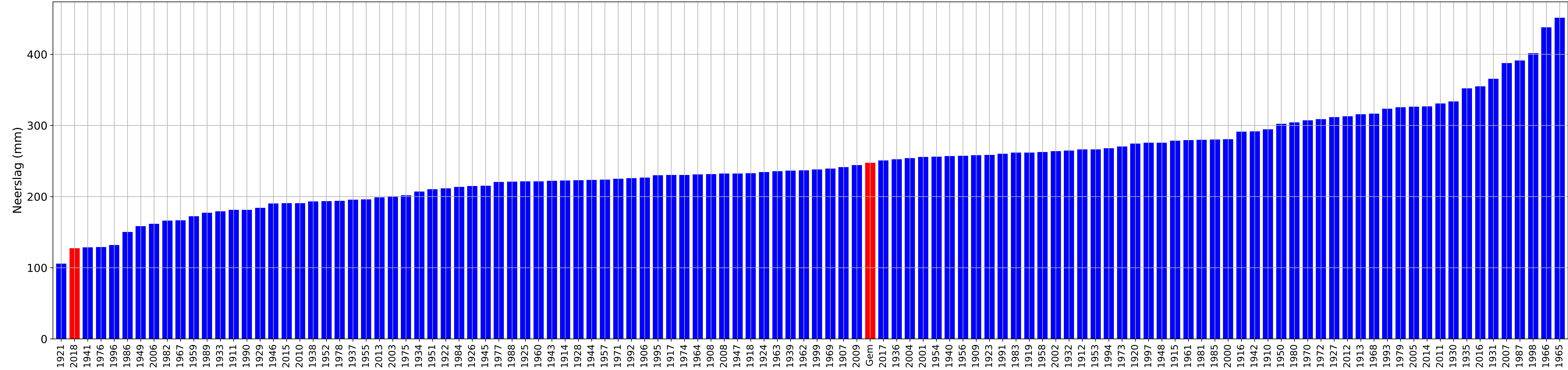
Totale neerslag per jaar van 01-04 t/m 31-07 voor De Bilt
